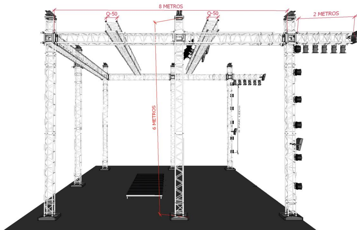
Vista Lateral
